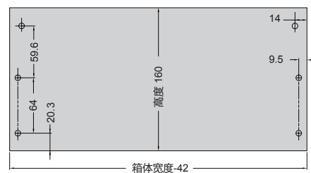
121铝薄帮方杆加高 背板开孔尺寸
